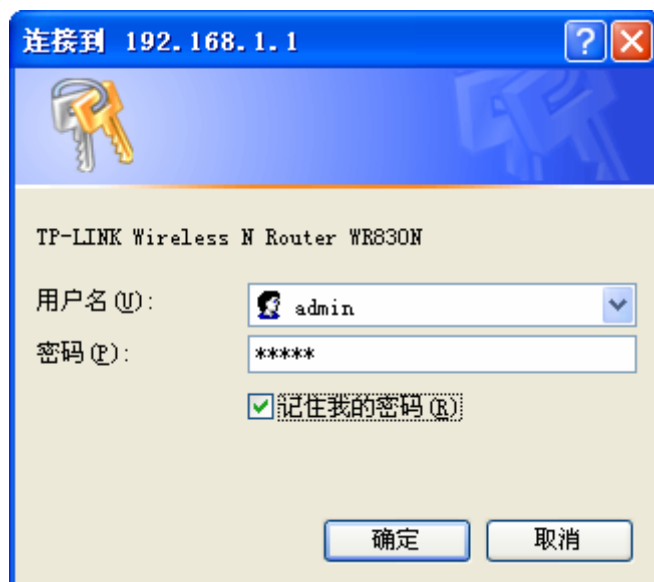
图 4-2 登录界面
