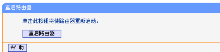
图 5-72 重启路由器
