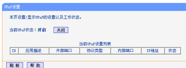
图 5-30 UPnP 设置
