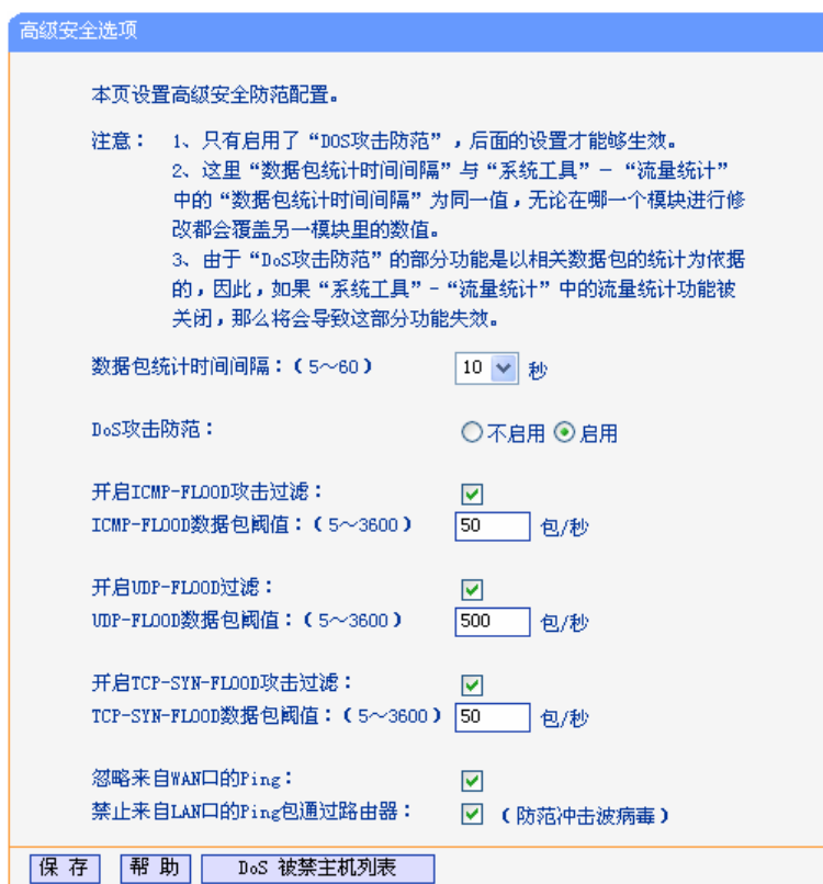
图 5-32 WAN 口 Ping
