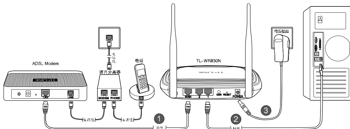
图 4-1 TL-WR830N 硬件安装示意图
